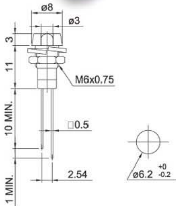
PLI-082 □ 00/ Direct
