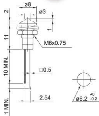
PLI-083 □ 00/ Diffuse
