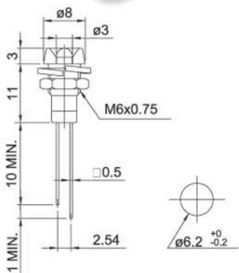
PLI-081 □ 00/ Reflect
